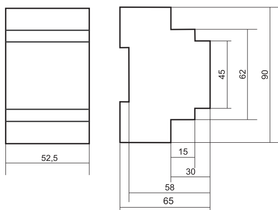
Рис.4 Габаритные размеры.
