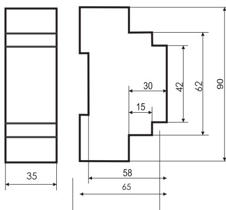
Рис.4 Габаритные размеры.
